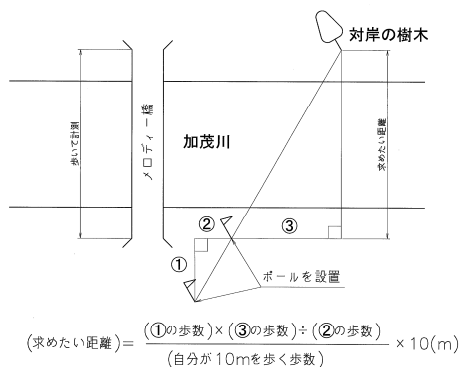
川幅計測説明図
